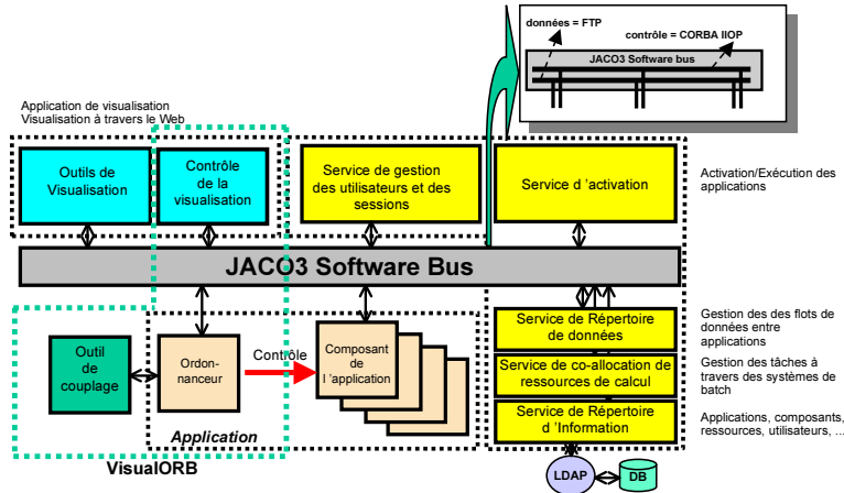
FIG. 2 – Environnement de simulation numérique distribuée JACO3
